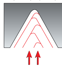
Боковое врезание с чередованием сторон профиля резьбы
