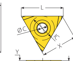
Тип On Edge – для наружной резьбы
