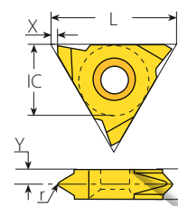
Тип V / пластины уменьшенной толщины
