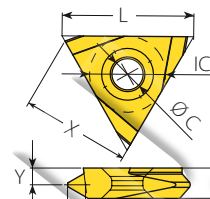
Тип On Edge
