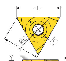
Тип On Edge – для внутренней резьбы
