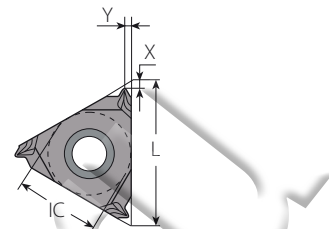
SCB со спеченным стружколомом
