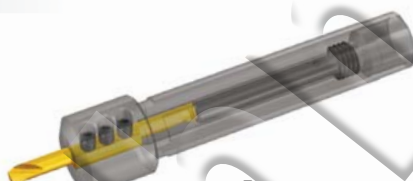
Держатели для двусторонних вставок Micro
