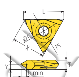
Тип On Edge
