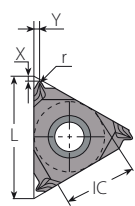
SCB со спеченным стружколомом
