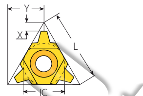
Тип U– для резьбы с крупным шагом
