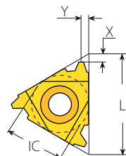
Базовый тип– для резьбы с крупным шагом
