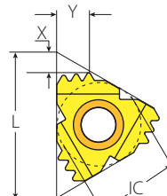
Тип F-Line M+
