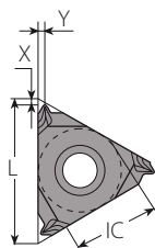
SCB со спеченным стружколомом
